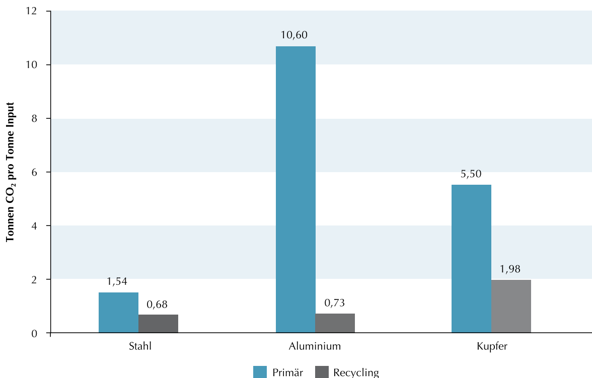
CO 2 -Emissionen von Primär- und Recyclingprozessen im Vergleich [5]
