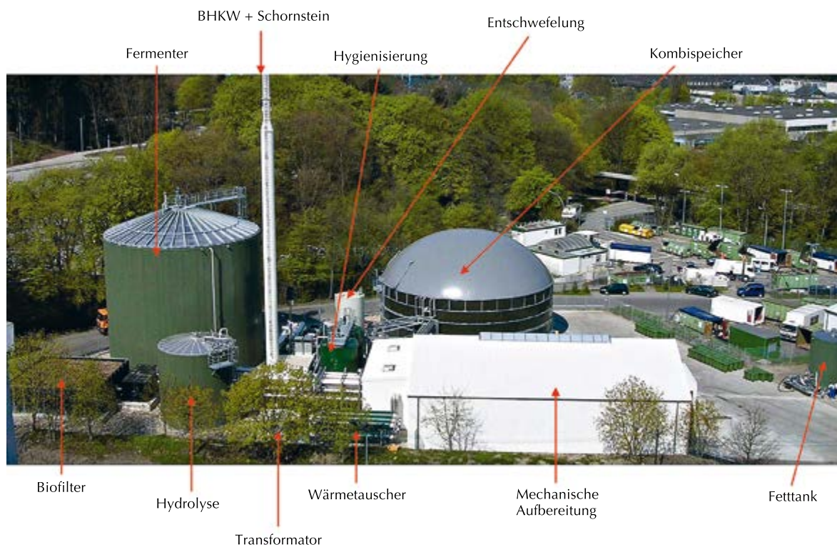
Nassvergärungsanlage („Biowerk“) in Hamburg-Stellingen
