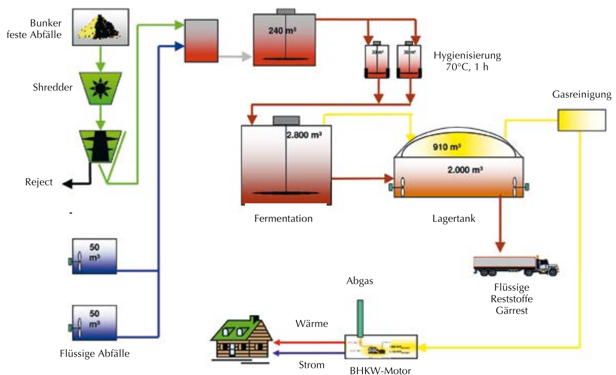
Ablaufschema der Nassvergärungsanlage in Hamburg-Stellingen
