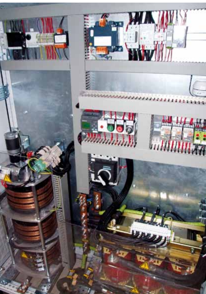
Der Spannungsstabilisator im Sportzentrum Bad Nenndorf
