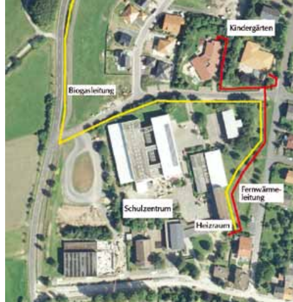
Biogasleitung und Fernwärmeleitung in Eiterfeld
