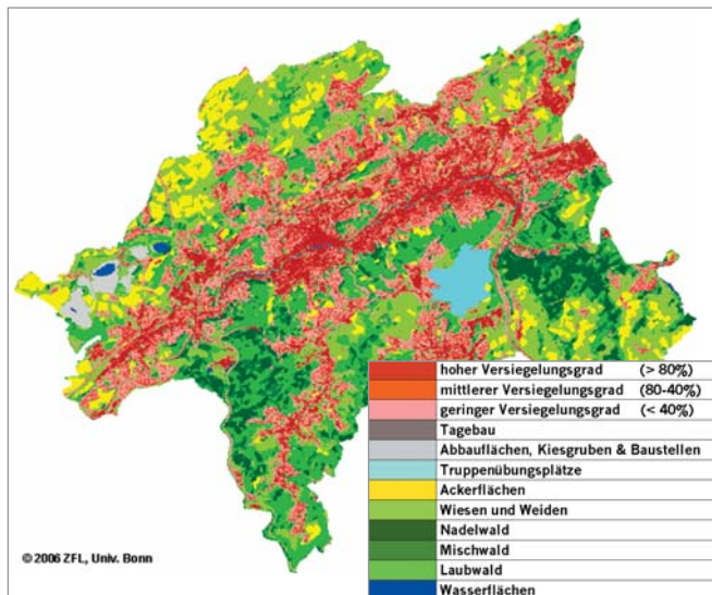
Klassifiziertes Satellitenbild einer Stadt: Versiegelungsgrade in Rottönen, Felder in gelb, Wald und Wiesen in grün (Quelle: vgl. Abb.)
