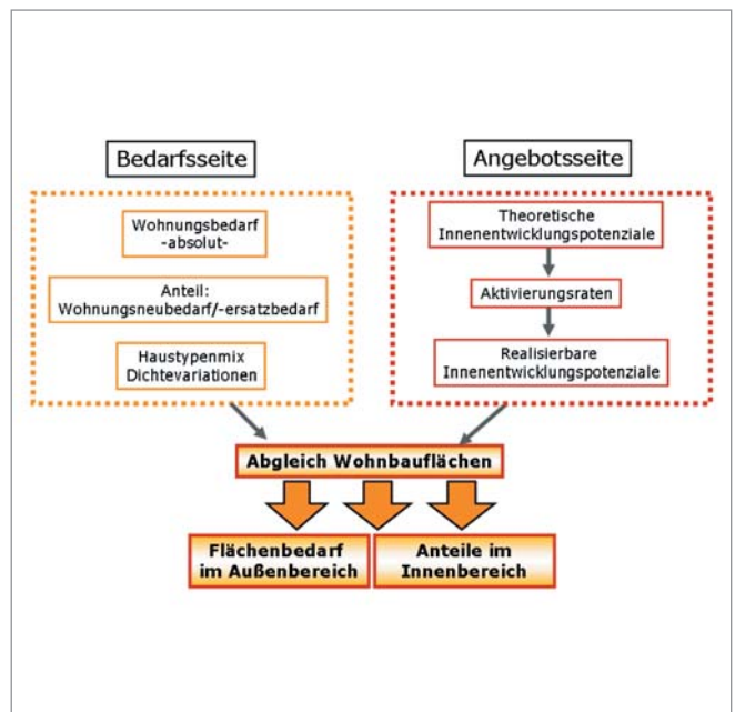
Methodisches Vorgehen bei komreg: Abgleich der Bedarfs- und Angebotsseite von Wohnbauflächen (Quelle: Öko-Institut)
