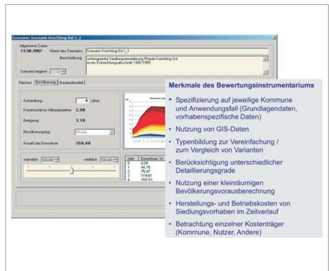
Merkmale des Bewertungsinstrumentariums in LEAN 2 (Quelle: ILS NRW/Planersocietät 2007)
