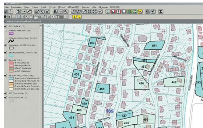
Baulandkataster Pfullingen (Bildschirmansicht): Erfassung von Nachverdichtungspotenzialen im Projekt „HAI“
