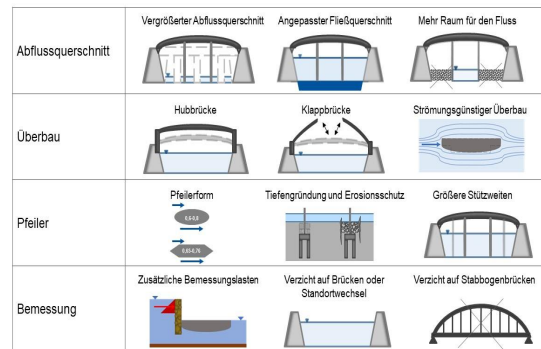
Abb. 24: Hochwasserangepasste Brückenbauweisen
